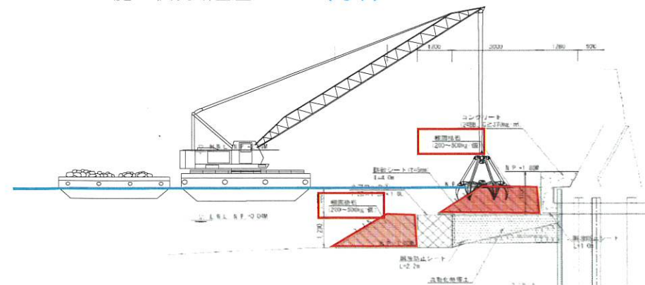
施工状況断面図 (海中)
