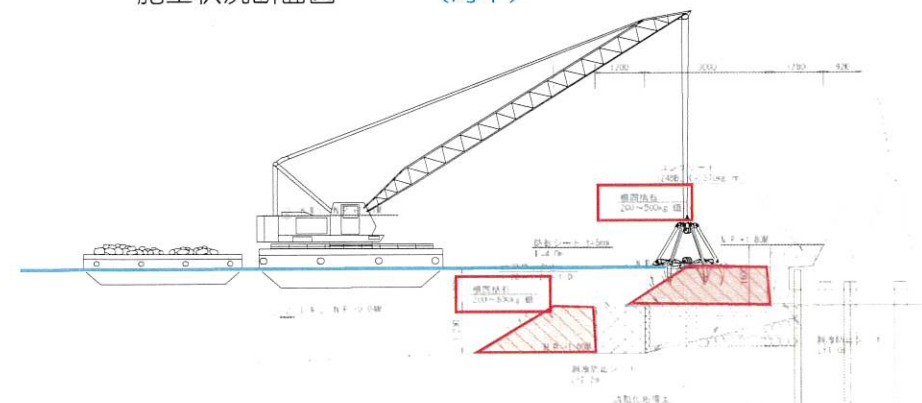
施工状況断面図 (海中)
